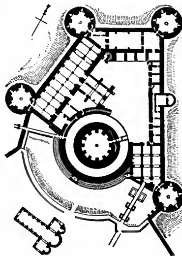
FIG. 7.—Coucy: Plan.
