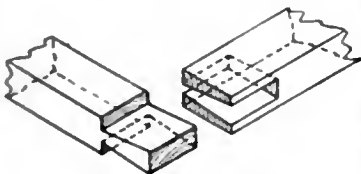
FIG. 8.—Dovetail.
