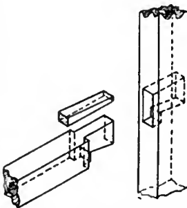
FIG. 15.—Dovetailed Tenon.
