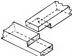
FIG. 10.—Halving.
