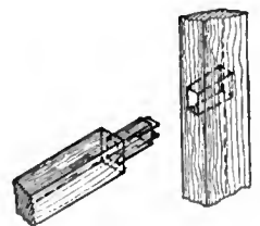
FIG. 18.—Foxtail Wedging.
